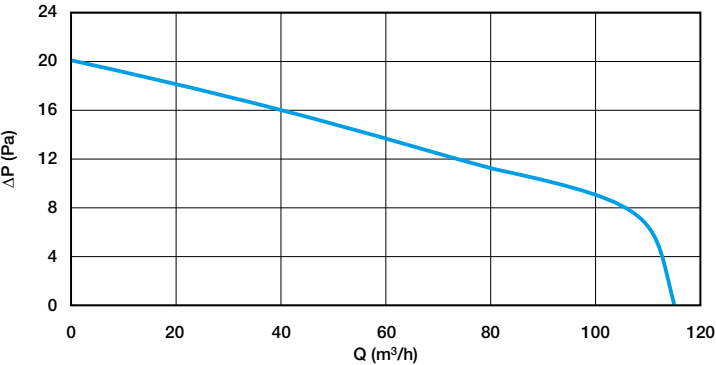
Curva aerúlica DECO 125
